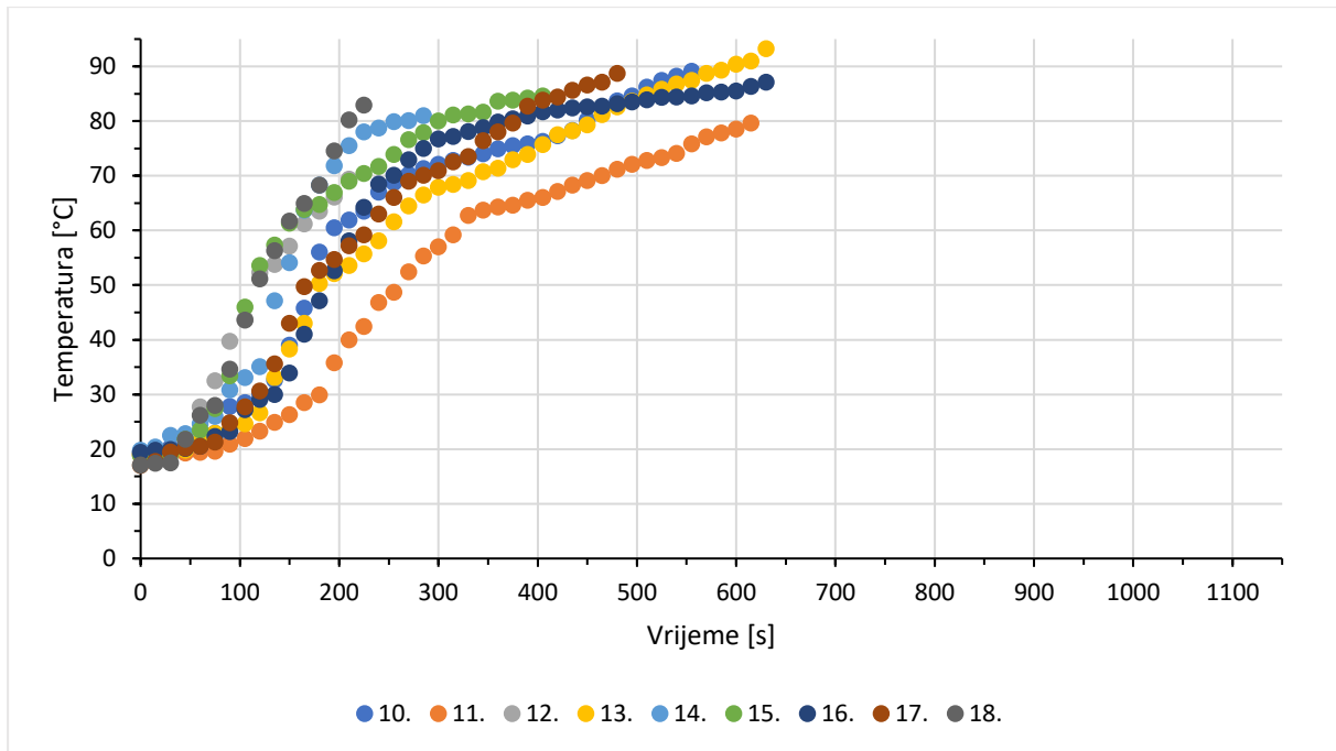
Slika 5.36 Dijagram ovisnosti maksimalne temperature o vremenu tijekom SPIF procesa (pokus 10.–18.)
