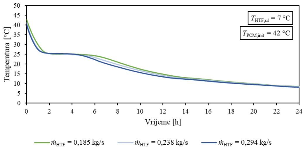
Slika 4.16. Vremenske promjene temperatura akumulatora topline prilikom korištenja topline dobivene eksperimentalnim mjerenjima na mjernoj poziciji T 2 za različite masene protoke fluida prijenosnika topline
