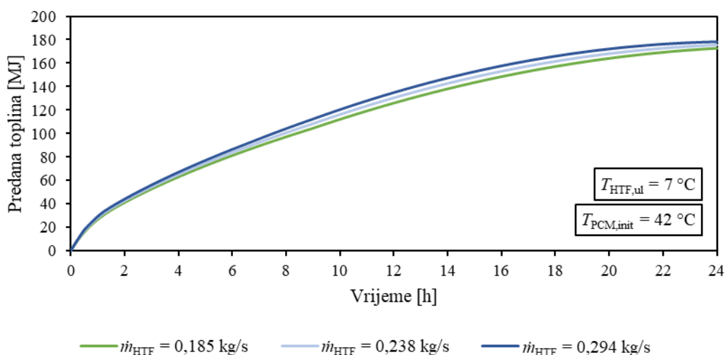
Slika 4.19. Vremenske promjene predanih toplina prilikom korištenja topline dobivene rezultatima eksperimentalnih mjerenja za različite masene protoke fluida prijenosnika topline
