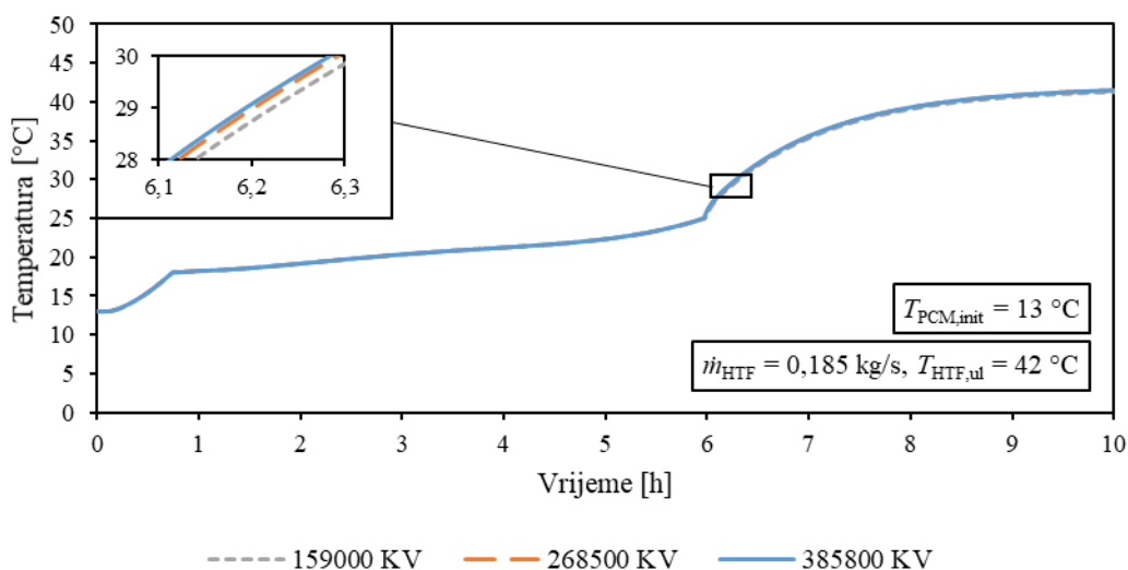
Slika 6.6. Vremenske promjene temperatura akumulatora topline prilikom taljenja na poziciji T_5 dobivene numeričkim proračunima za različite gustoće mreže
