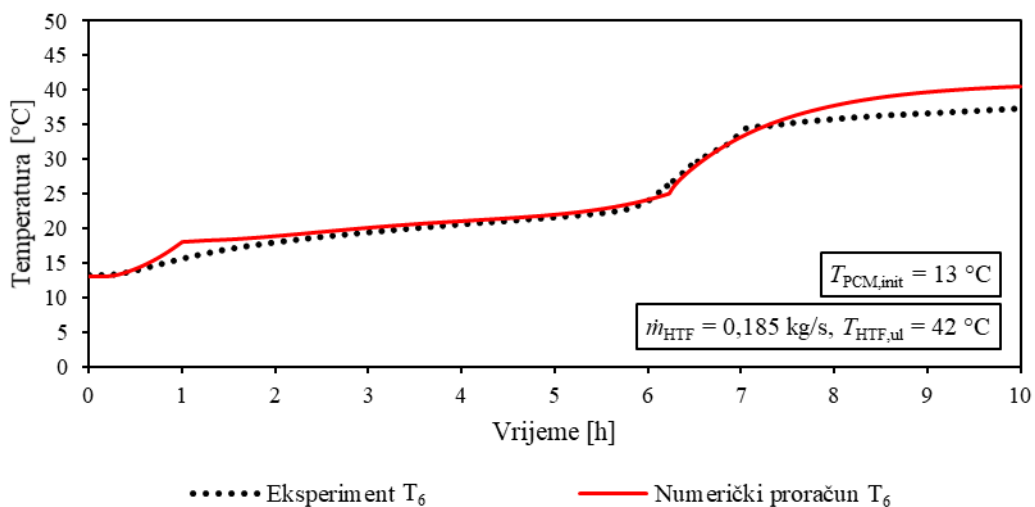
Slika 7.2. Vremenske promjene temperatura akumulatora topline prilikom taljenja dobivene eksperimentalno i numerički na poziciji T_6
