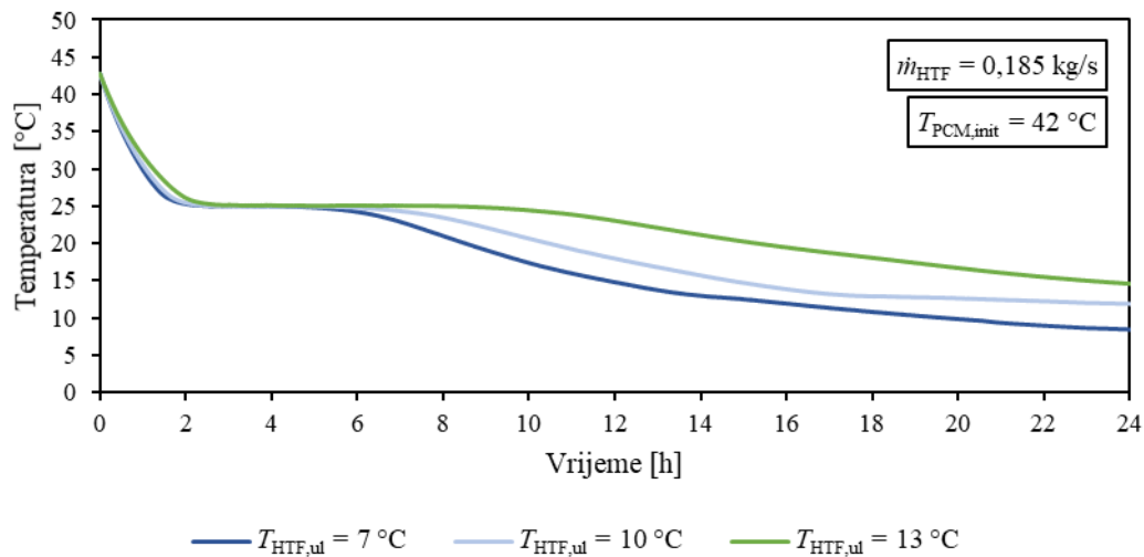
Slika 4.6. Vremenske promjene temperatura akumulatora topline prilikom korištenja topline dobivene eksperimentalnim mjerenjima na mjernoj poziciji T 2 za različite ulazne temperature fluida prijenosnika topline
