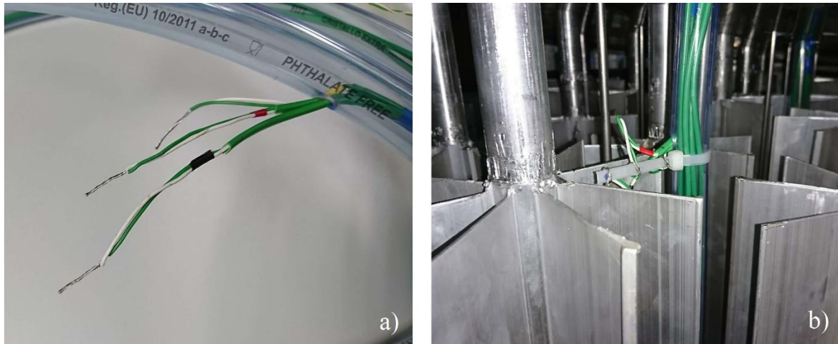
Slika 3.8. Postavljanje mjernih osjetnika u latentni spremnik topline, a) termoparovi u gumenoj cijevi, b) termoparovi učvršćeni plastičnim vezicama na pozicijama oko cijevi
