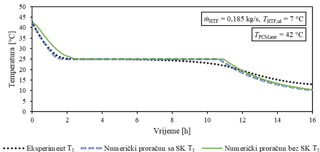
Slika 7.10. Vremenske promjene temperatura akumulatora topline prilikom skrućivanja dobivene eksperimentalno i numerički s i bez utjecaja slobodne konvekcije na poziciji T 5
