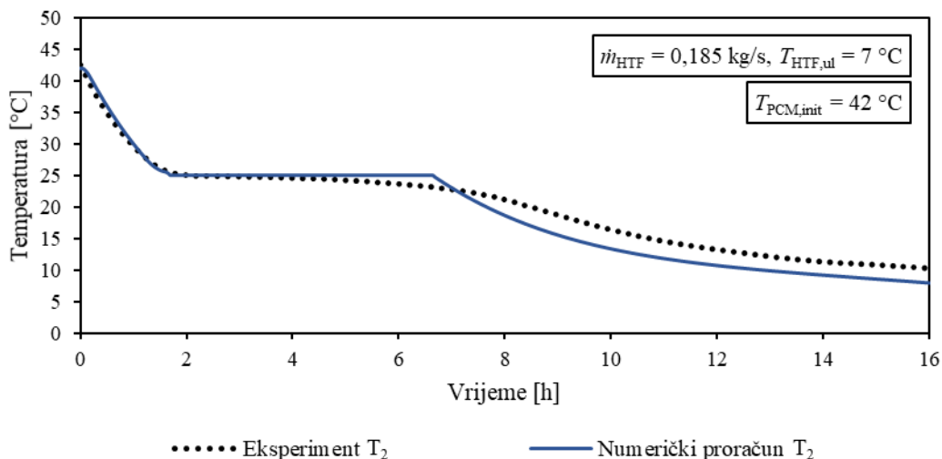
Slika 7.3. Vremenske promjene temperatura akumulatora topline prilikom skrućivanja dobivene eksperimentalno i numerički na poziciji T 2
