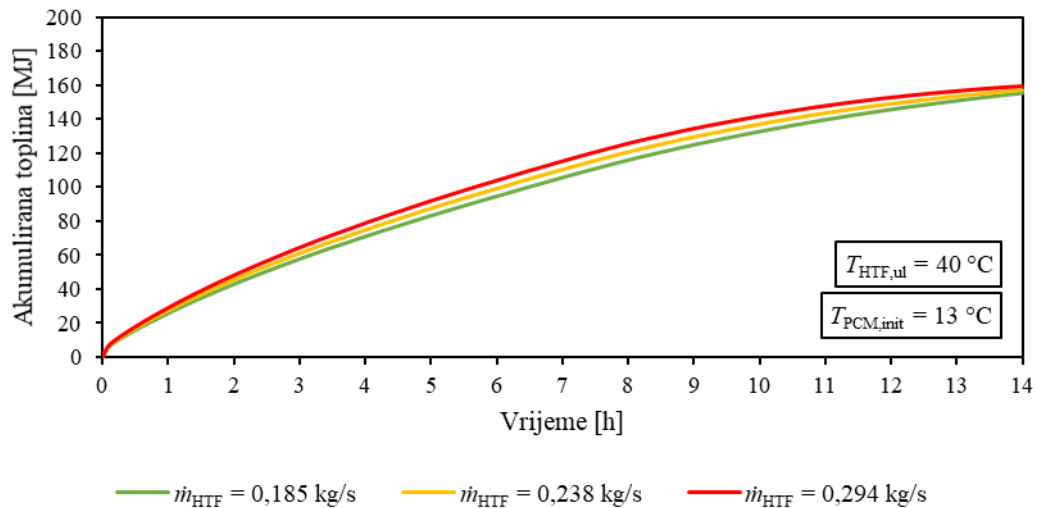
Slika 4.14. Vremenske promjene akumuliranih toplina prilikom spremanja topline dobivene rezultatima eksperimentalnih mjerenja za različite masene protoke fluida prijenosnika topline
