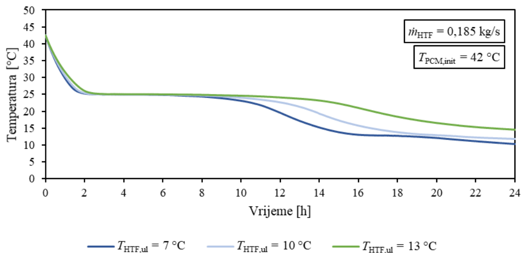
Slika 4.7. Vremenske promjene temperatura akumulatora topline prilikom korištenja topline dobivene eksperimentalnim mjerenjima na mjernoj poziciji T 5 za različite ulazne temperature fluida prijenosnika topline
