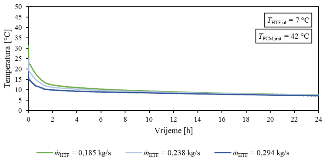
Slika 4.18. Vremenske promjene izlaznih temperatura fluida prijenosnika topline prilikom korištenja topline dobivene eksperimentalnim mjerenjima za različite masene protoke fluida prijenosnika topline
