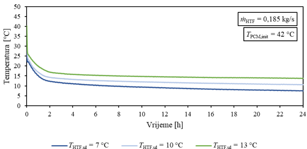
Slika 4.8. Vremenske promjene izlaznih temperatura fluida prijenosnika topline prilikom korištenja topline dobivene eksperimentalnim mjerenjima za različite ulazne temperature fluida prijenosnika topline
