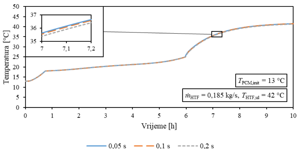
Slika 6.7. Vremenske promjene temperatura akumulatora topline prilikom taljenja na poziciji T_5 dobivene numeričkim proračunima za različite vremenske korake
