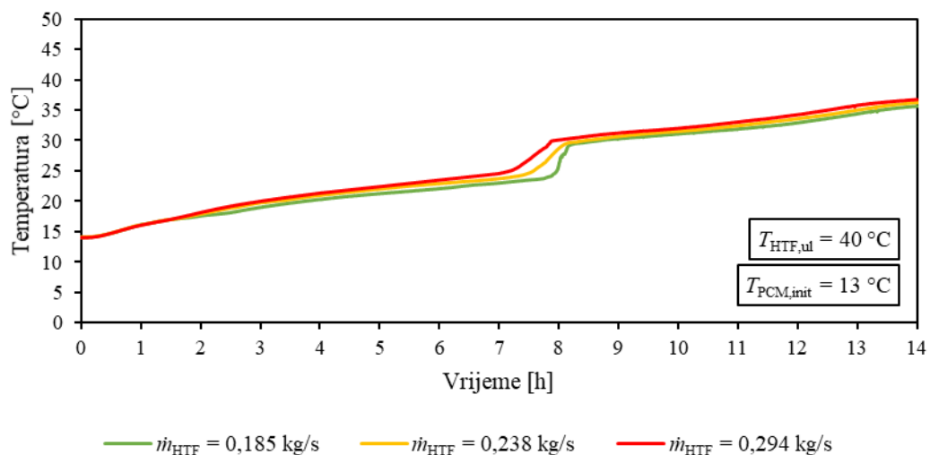
Slika 4.11. Vremenske promjene temperatura akumulatora topline prilikom spremanja topline dobivene eksperimentalnim mjerenjima na mjernoj poziciji T 6 za različite masene protoke fluida prijenosnika topline
