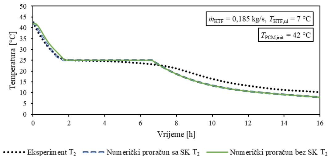
Slika 7.9. Vremenske promjene temperatura akumulatora topline prilikom skrućivanja dobivene eksperimentalno i numerički s i bez utjecaja slobodne konvekcije na poziciji T 2
