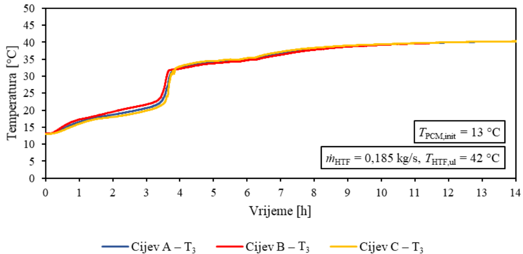
Slika 3.9. Vremenske promjene temperatura akumulatora topline prilikom taljenja na poziciji T_3 dobivene eksperimentalnim mjerenjima na različitim cijevima
