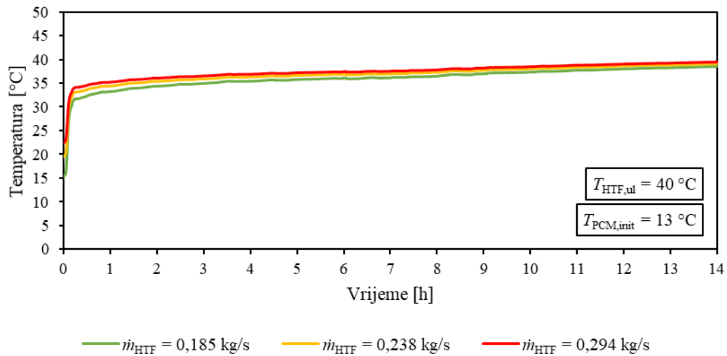
Slika 4.13. Vremenske promjene izlaznih temperatura fluida prijenosnika topline prilikom spremanja topline dobivene eksperimentalnim mjerenjima za različite masene protoke fluida prijenosnika topline
