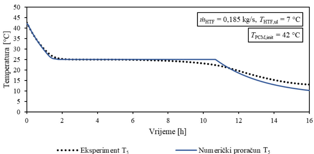
Slika 7.4. Vremenske promjene temperatura akumulatora topline prilikom skrućivanja dobivene eksperimentalno i numerički na poziciji T 5
