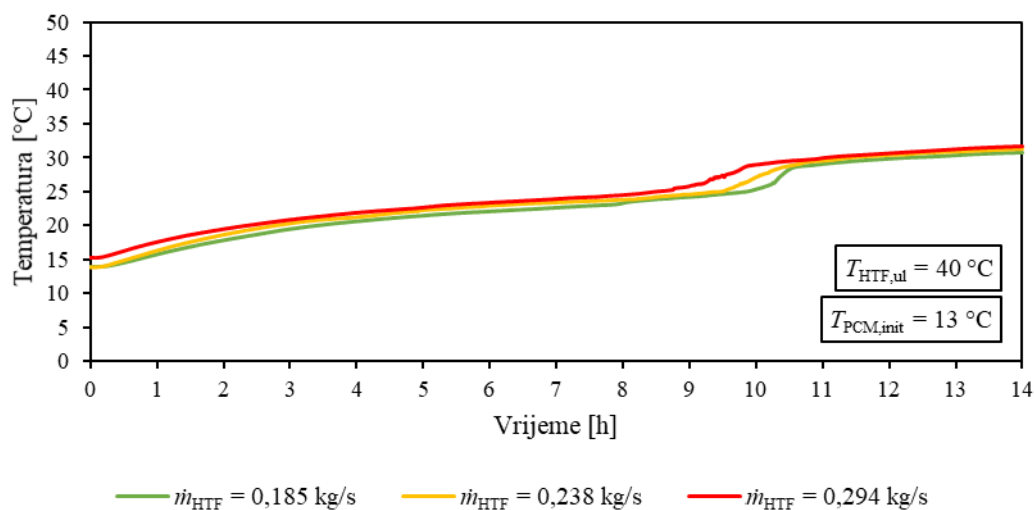
Slika 4.12. Vremenske promjene temperatura akumulatora topline prilikom spremanja topline dobivene eksperimentalnim mjerenjima na mjernoj poziciji T_9 za različite masene protoke fluida prijenosnika topline
