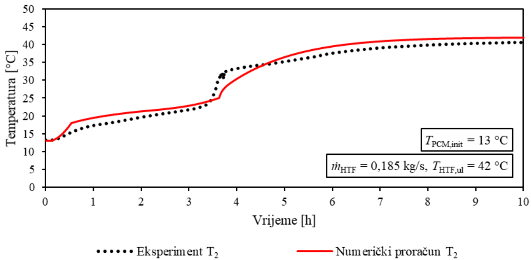
Slika 7.1. Vremenske promjene temperatura akumulatora topline prilikom taljenja dobivene eksperimentalno i numerički na poziciji T_2
