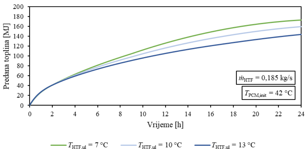
Slika 4.9. Vremenske promjene predanih toplina prilikom korištenja topline dobivene rezultatima eksperimentalnih mjerenja za različite ulazne temperature fluida prijenosnika topline
