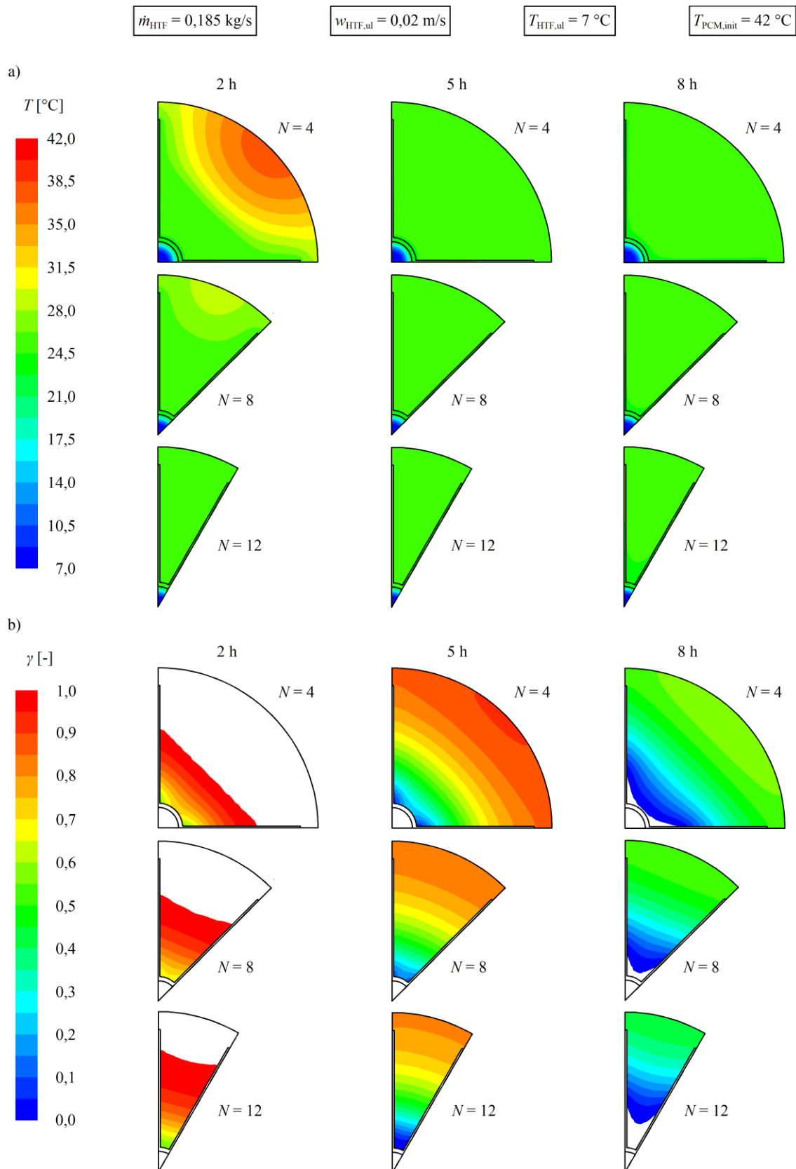
Slika 8.5. Usporedba raspodjela temperatura i udjela kapljevite faze u ravnini xy za z = 0,75 m prilikom korištenja topline dobivenih numeričkim proračunima u proračunskim vremenima 2, 5 i 8 h za konfiguracije latentnog spremnika topline s 4, 8 i 12 lamela
