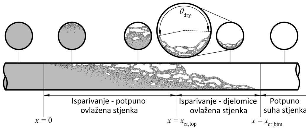
Slika 3.23 Promjene režima strujanja tijekom strujanja s vrenjem CO_2
