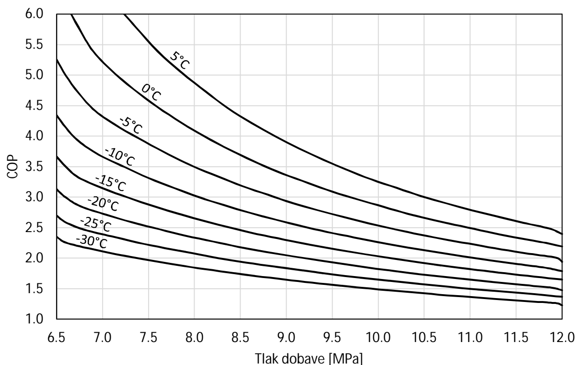
Slika 6.3 Linije optimalnih COP pri različitim temperaturama isparivanja
