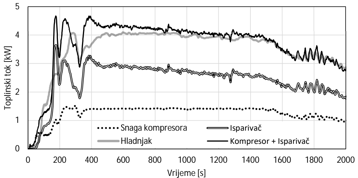
Slika 5.25 Tokovi energije u izmjenjivačima i kompresoru
