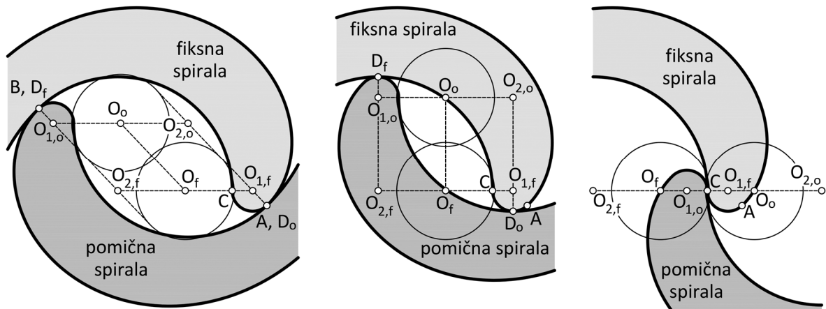
Slika 3.17 Početak (lijevo) i kraj (desno) dodira kružnih lukova
