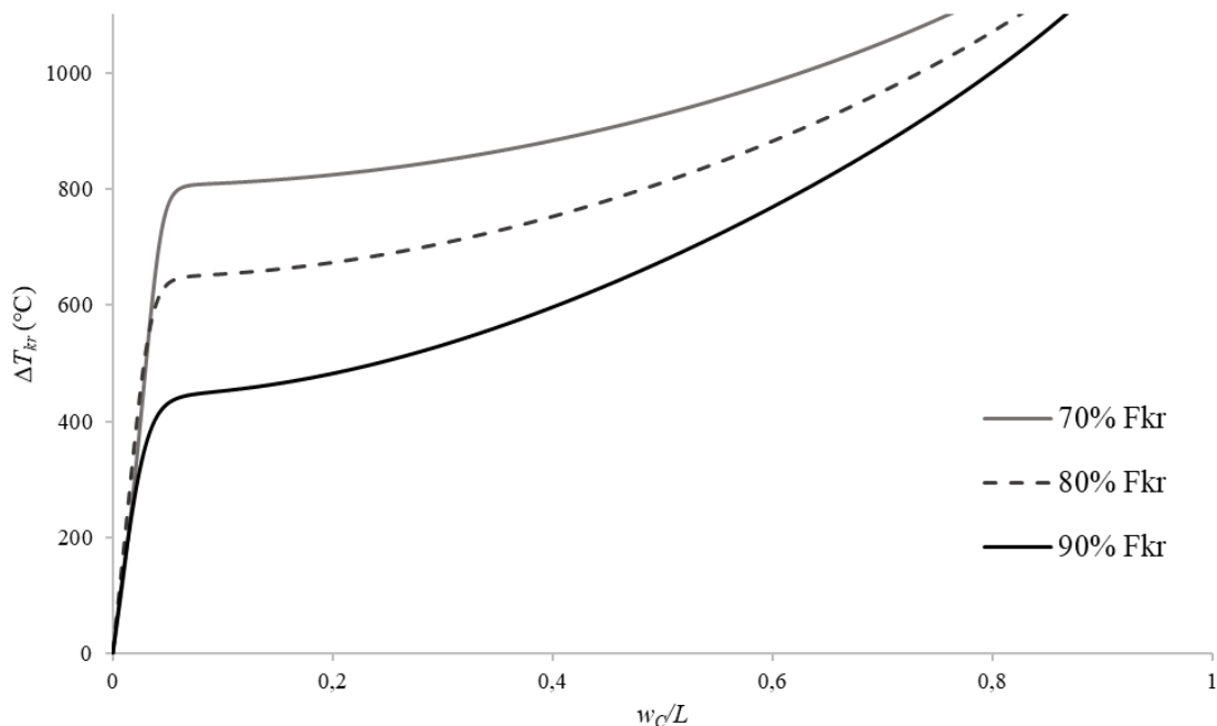
Sl. 5.55 Uz primjer 9: Dijagram temperatura-pomak za tri razine kritične sile F (+) za p = 0,5 , LTR
