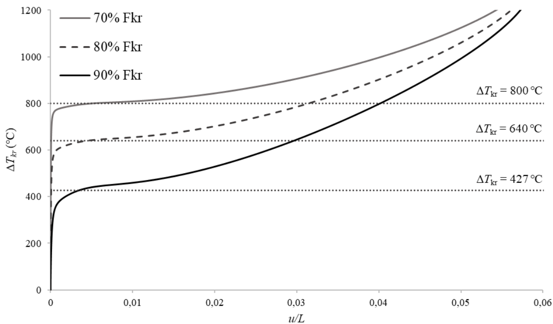
Sl. 5.46 Uz primjer 8: Dijagram temperatura-pomak, torzijsko-fleksijsko izvijanje C-profila za p = 1
