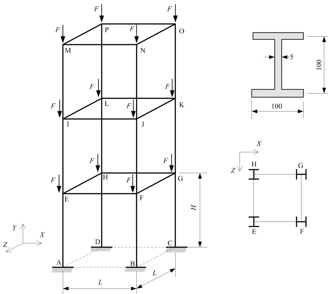
Sl. 5.59 Uz primjer 10: Prostorni okvir opterećen vertikalnim silama inteziteta F
