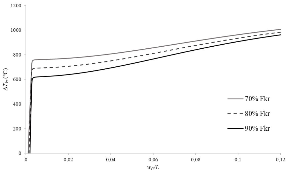
Sl. 5.56 Uz primjer 9: Dijagram temperatura-pomak za tri razine kritične sile F (-) za p = 0 , UTR
