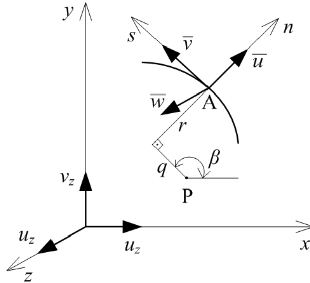
Sl. 3.1 Pomaci točaka konture poprečnog presjeka
