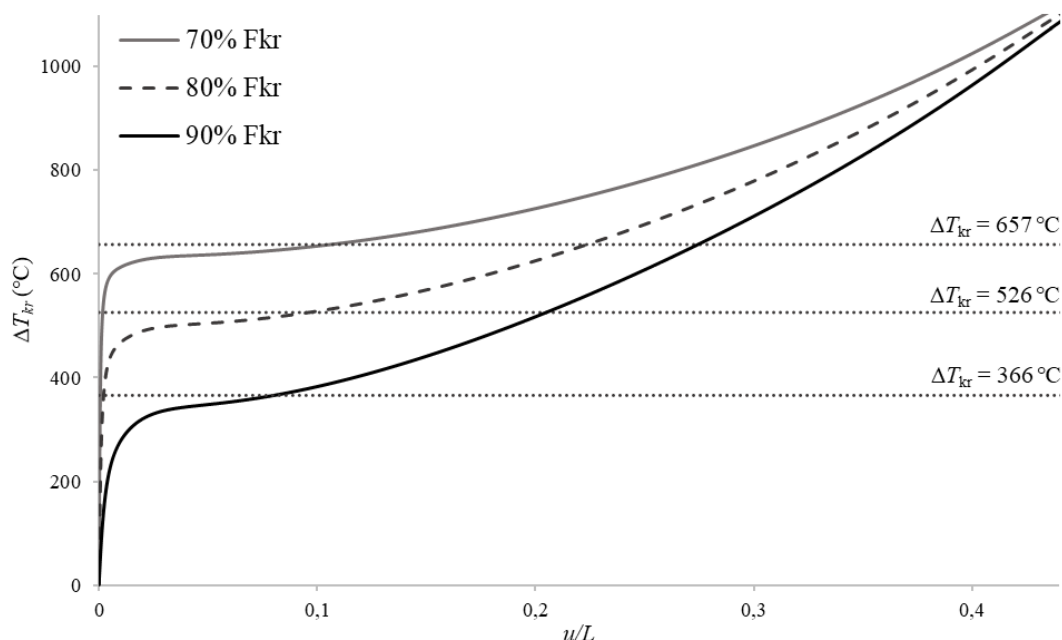
Sl. 5.39 Uz primjer 8: Dijagram temperatura-pomak, torzijsko-fleksijsko izvijanje I-profila za p = 0
