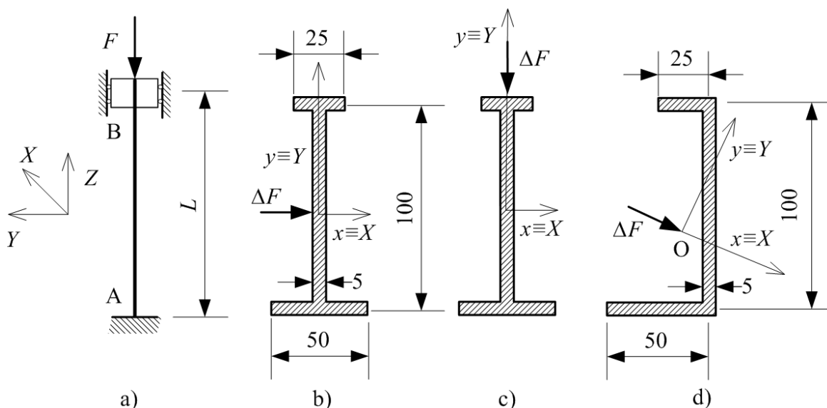
Sl. 5.38 Uz primjer 8: a) Tlačno opterećen stup uklješten na oba kraja; b) torzijsko-fleksijsko izvijanje monosimetričnog I-profila (I1); c) fleksijsko izvijanje monosimetričnog I-profila (I2); d) torzijsko fleksijsko izvijanje nesimetričnog C-profila
