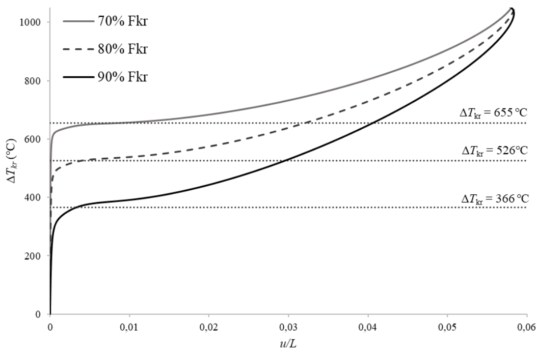
Sl. 5.45 Uz primjer 8: Dijagram temperatura-pomak, torzijsko-fleksijsko izvijanje C-profila za p = 0
