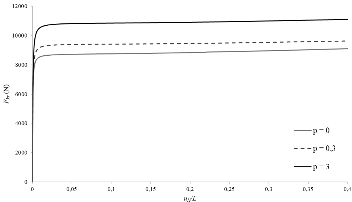
Sl. 5.62 Uz primjer 10: Nelinearni odziv sway oblika izvijanja
