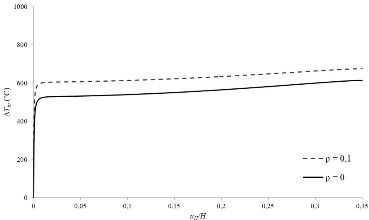
Sl. 5.64 Uz primjer 10: Usporedba savršenog i poroznog materijala za eksponent p = 0,3 pri 80% F_{kr} , UTR
