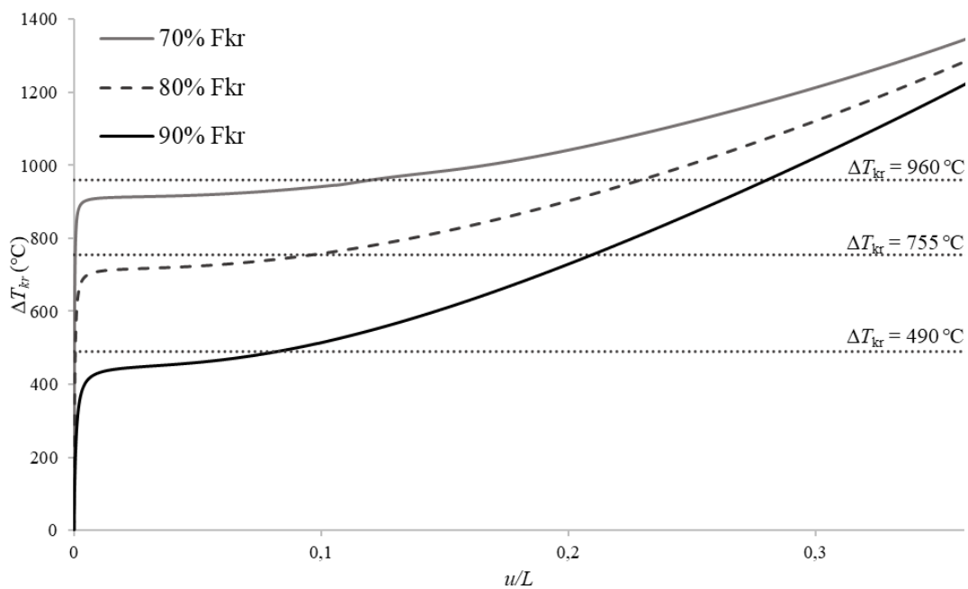
Sl. 5.44 Uz primjer 8: Dijagram temperatura-pomak, fleksijsko izvijanje I-profila za p = 5
