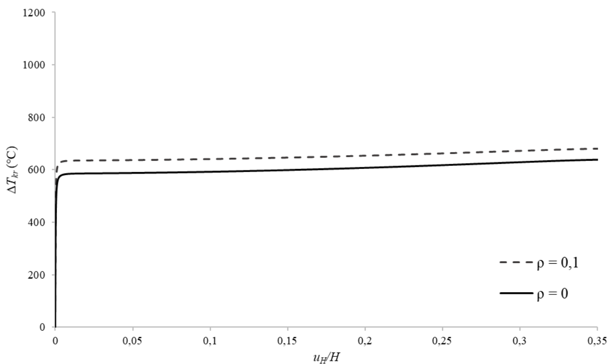
Sl. 5.68 Uz primjer 10: Usporedba savršenog i poroznog materijala za eksponent p = 3 pri 70% F_{kr} , LTR
