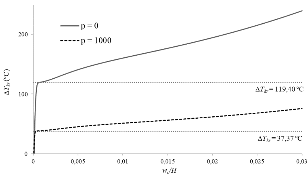
Sl. 5.13 Uz primjer 3: Dijagram temperatura-pomak za izotropne materijale, UTR
