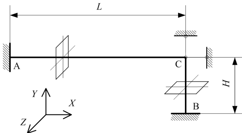
Sl. 5.12 Uz primjer 3: L – okvir
