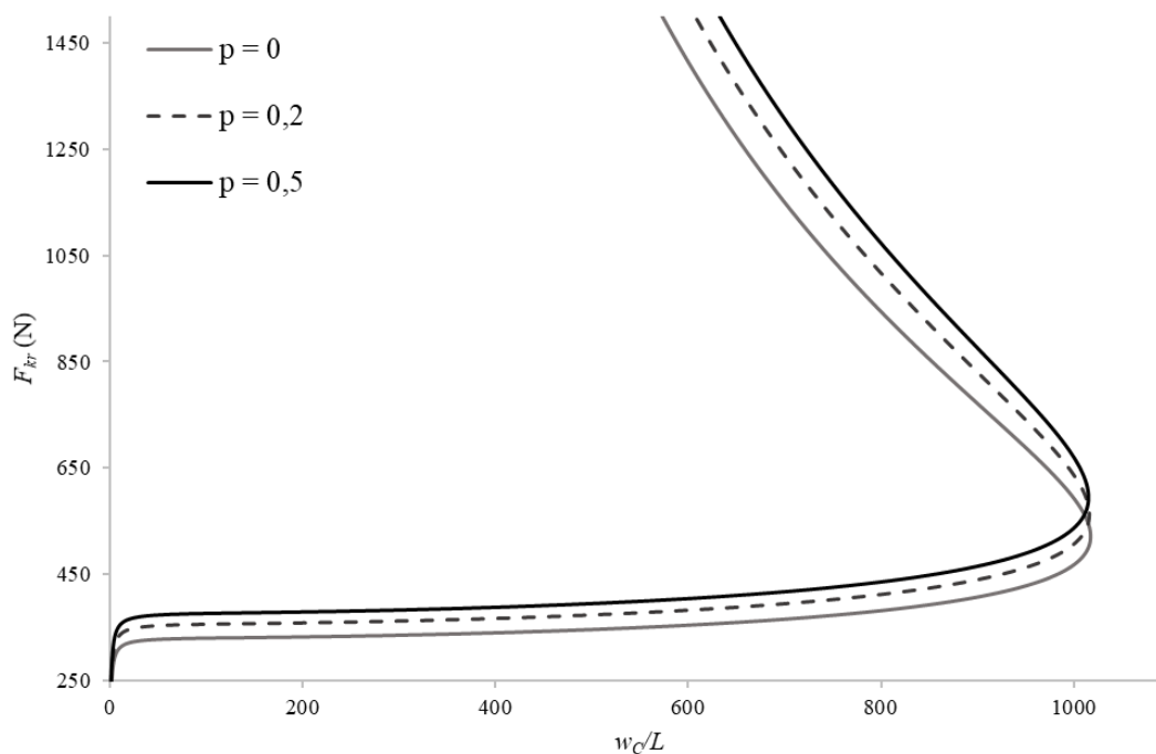
Sl. 5.49 Uz primjer 9: Dijagram sila-pomak za različite eksponente p : a) kritična faza; b) postkritična faza
