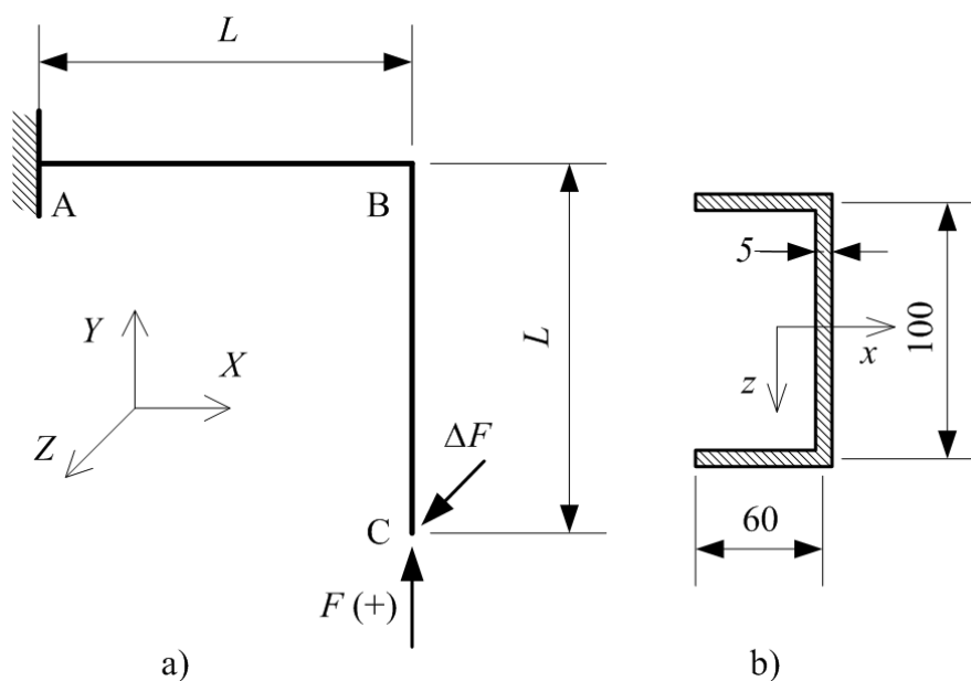
Sl. 5.48 Uz primjer 9: a) L-okvir; b) monosimetričan C-profil
