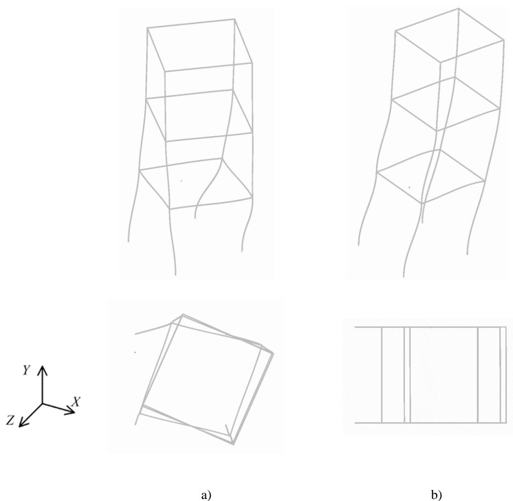
Sl. 5.60 Uz primjer 10: a) twist-sway oblik izvijanja; b) sway oblik izvijanja
