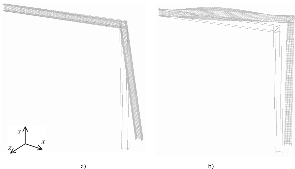
Sl. 5.50 Uz primjer 9: Shell model izvijanja L-okvira pri: a) F(+) , b) F(-)
