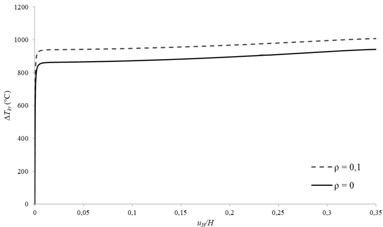
Sl. 5.65 Uz primjer 10: Usporedba savršenog i poroznog materijala za eksponent p = 3 pri 70% F_{kr} , UTR
