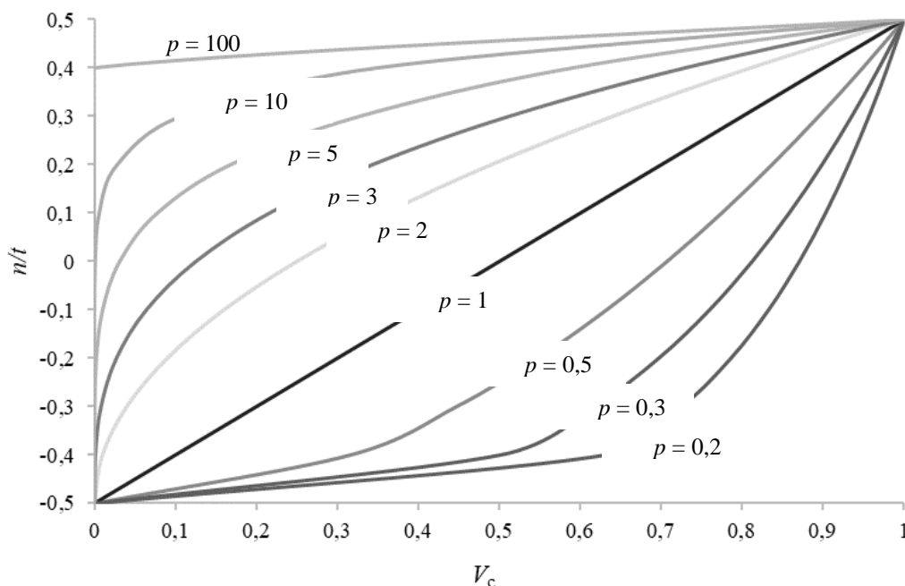
Sl. 2.4 Volumni udio keramike po stijenci poprečnog presjeka
