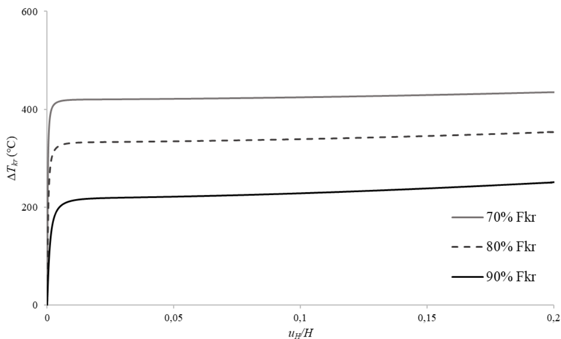
Sl. 5.66 Uz primjer 10: Dijagram temperatura-pomak za tri razine kritične sile F za p = 0 , LTR
