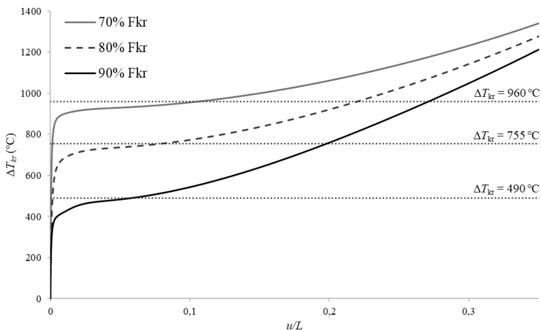
Sl. 5.41 Uz primjer 8: Dijagram temperatura-pomak, torzijsko-fleksijsko izvijanje I-profila za p = 5
