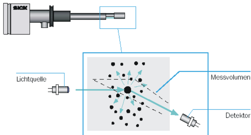
S. 23.3. Princip rada analizatora
