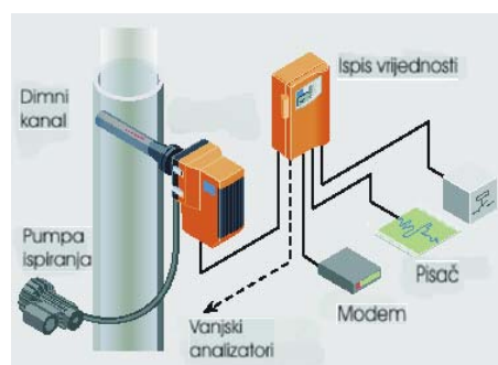
UV spektroskopija
