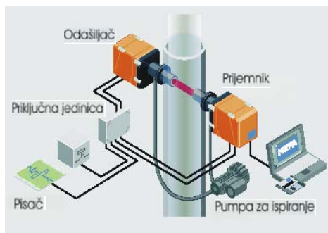
Apsorpcija IC zračenja
