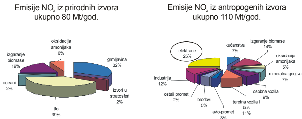
Sl. 21.4 Globalna godišnja emisija NO x
