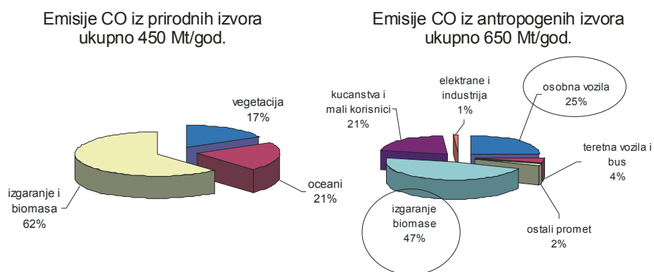
Sl. 21.3. Globalna godišnja emisija CO
