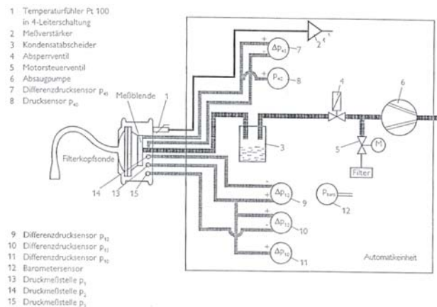
Sonda uređaja i priključci za mjerenja
