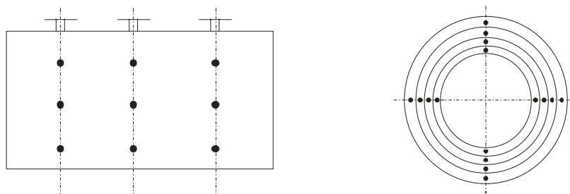
mjerne točke kod pravokutnog presjeka mjerne točke kod kružnog presjeka
