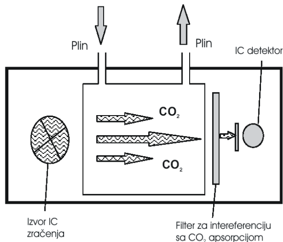
Sl. 22. 3 Senzor na principu IC apsorpcije
